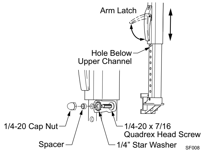
Figure 8. Stop Bolt.
